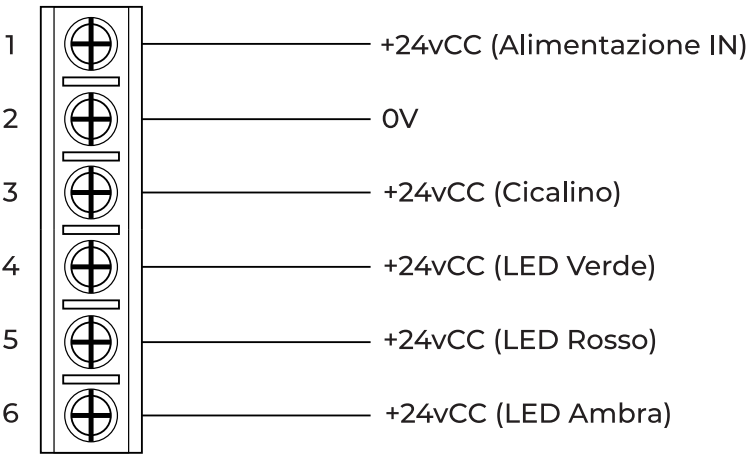
Schema di Cablaggio 1 (CC)
