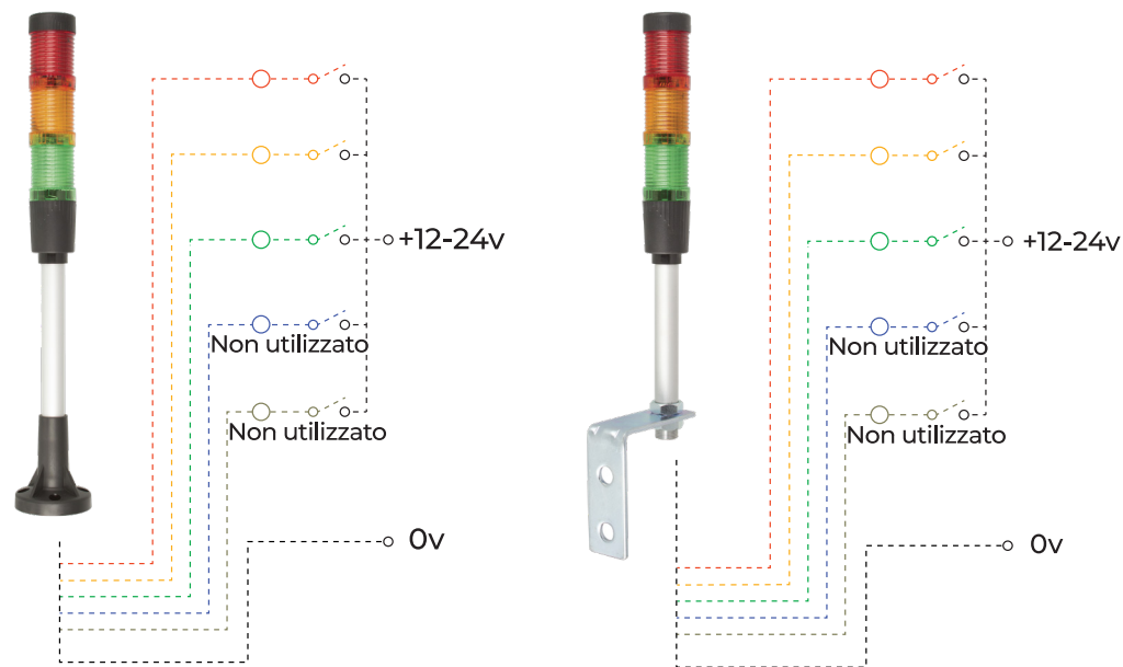
Schema di Cablaggio 1 (FT100)
