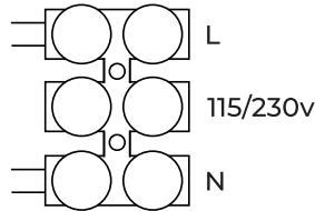
Diagrama eléctrico 2
