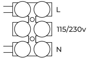
Schaltplan 2
