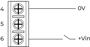
Schéma câblage 1 (Vcc)
