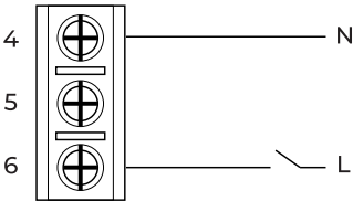
Schéma câblage 2 (Vca)
