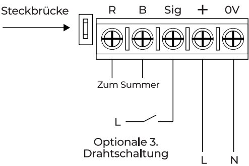
Schaltplan 2 (AC)
