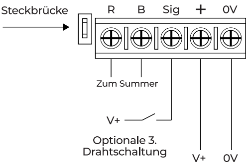
Schaltplan 1 (DC)
